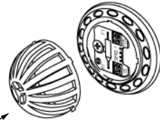
Lämpötilatunnistin ylikuumenemissuojalla
